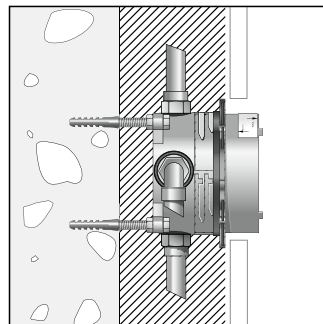
Szerelés fal elé, itt távtartókkal és M 10 méretű töcsavarokkal
