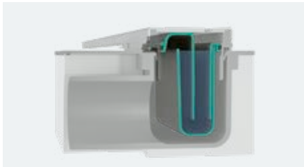
Hagyományos szifonos technológia
