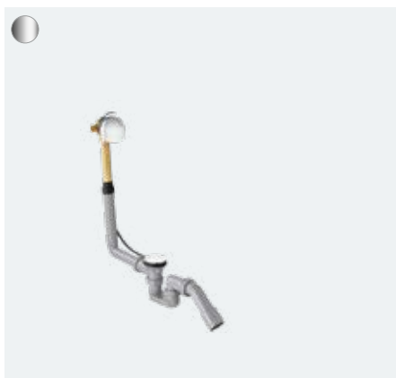
Exafill komplett készlet kádőtöltővel komplett készlet le- és túlfolyó garnitúrával, normál kádakhoz # 58123, -000
