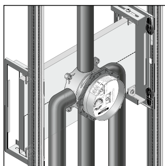
Szerelés tartórendszerre
