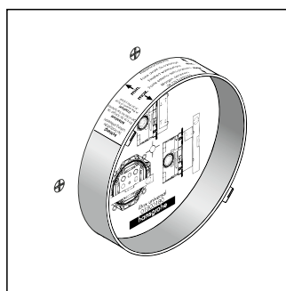
Szerelés készház szerelőlapokra vagy készcellákra
