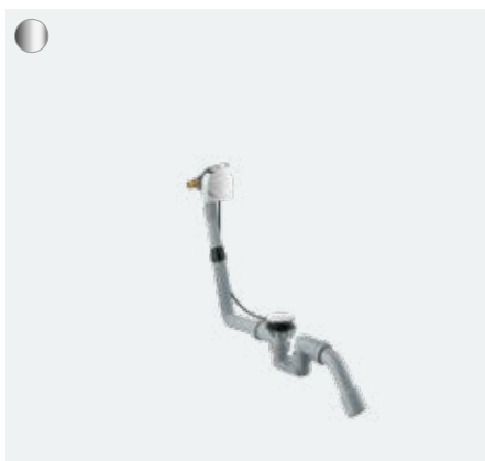
Exafill S komplett készlet kádőtöltővel le- és túlfolyó garnitúrával, normál kádakhoz # 58113, -000
