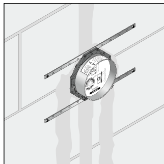
Szerelés szerelősin készlettel
